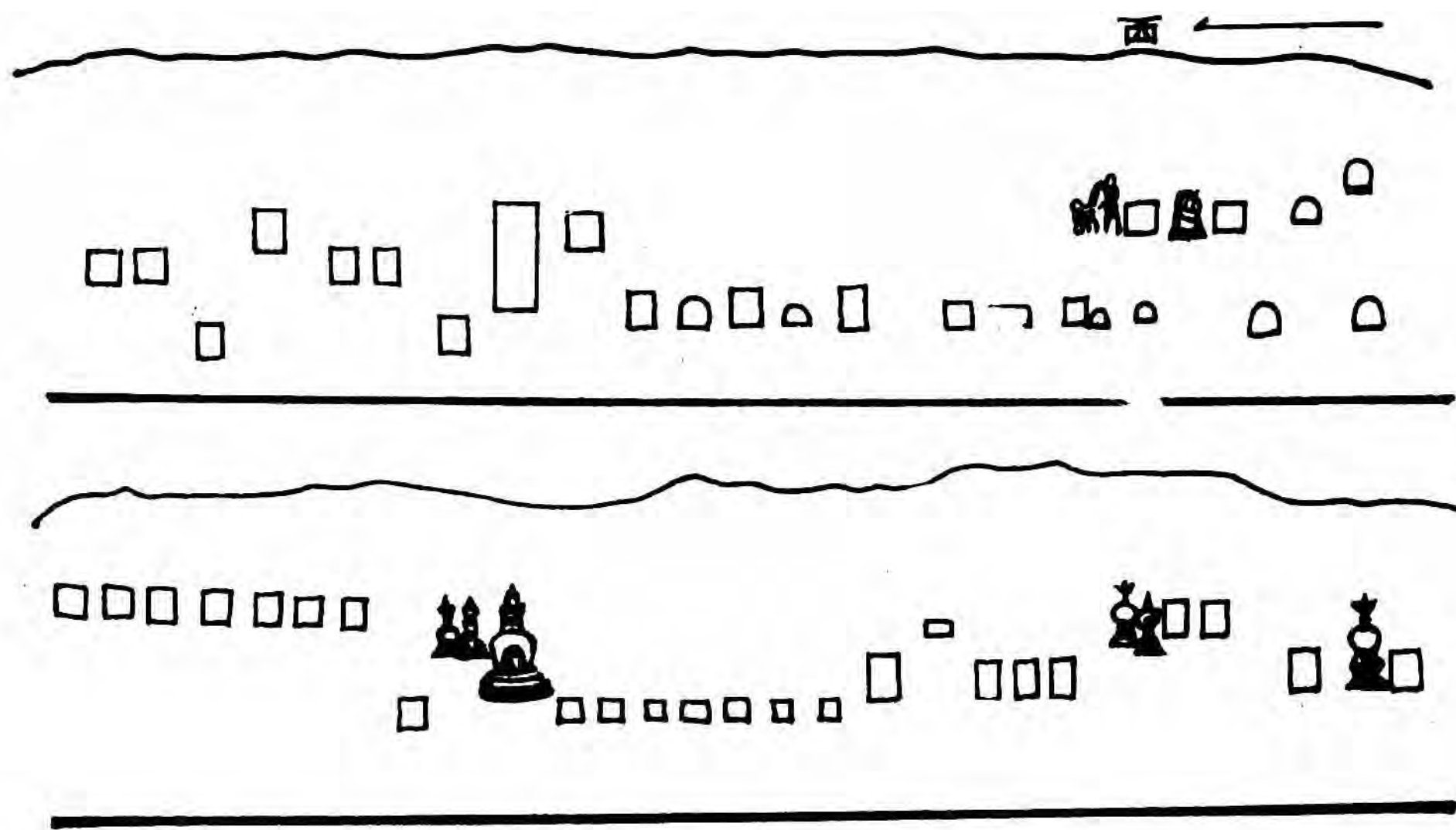
百眼窑石窟寺平面图
